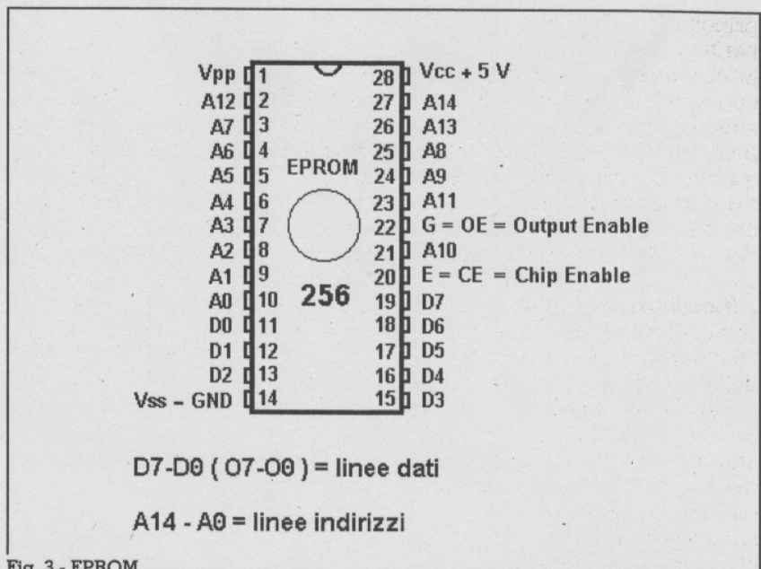
Fig. 3 - EPROM
